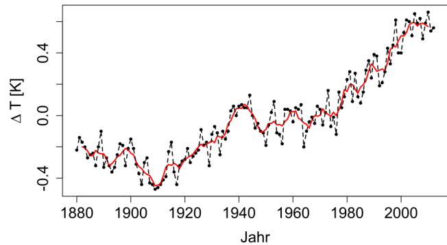
Globale Oberflächentemperaturen (Ref. 1951-80)
